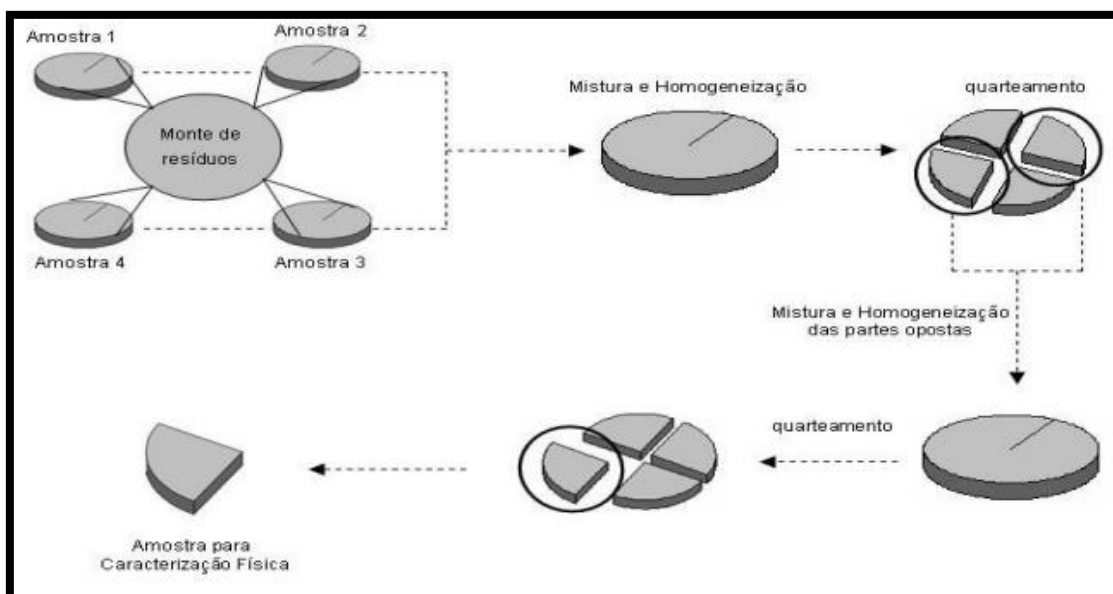
Figura 31 – Diagrama do processo de quarteamento dos resíduos sólidos
