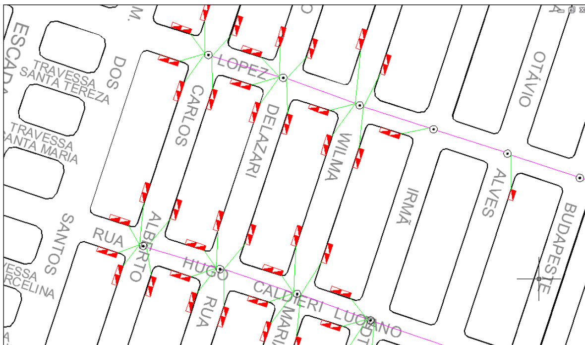
Figura 49 - Detalhe do Mapa de Cadastramento do Sistema de Drenagem
