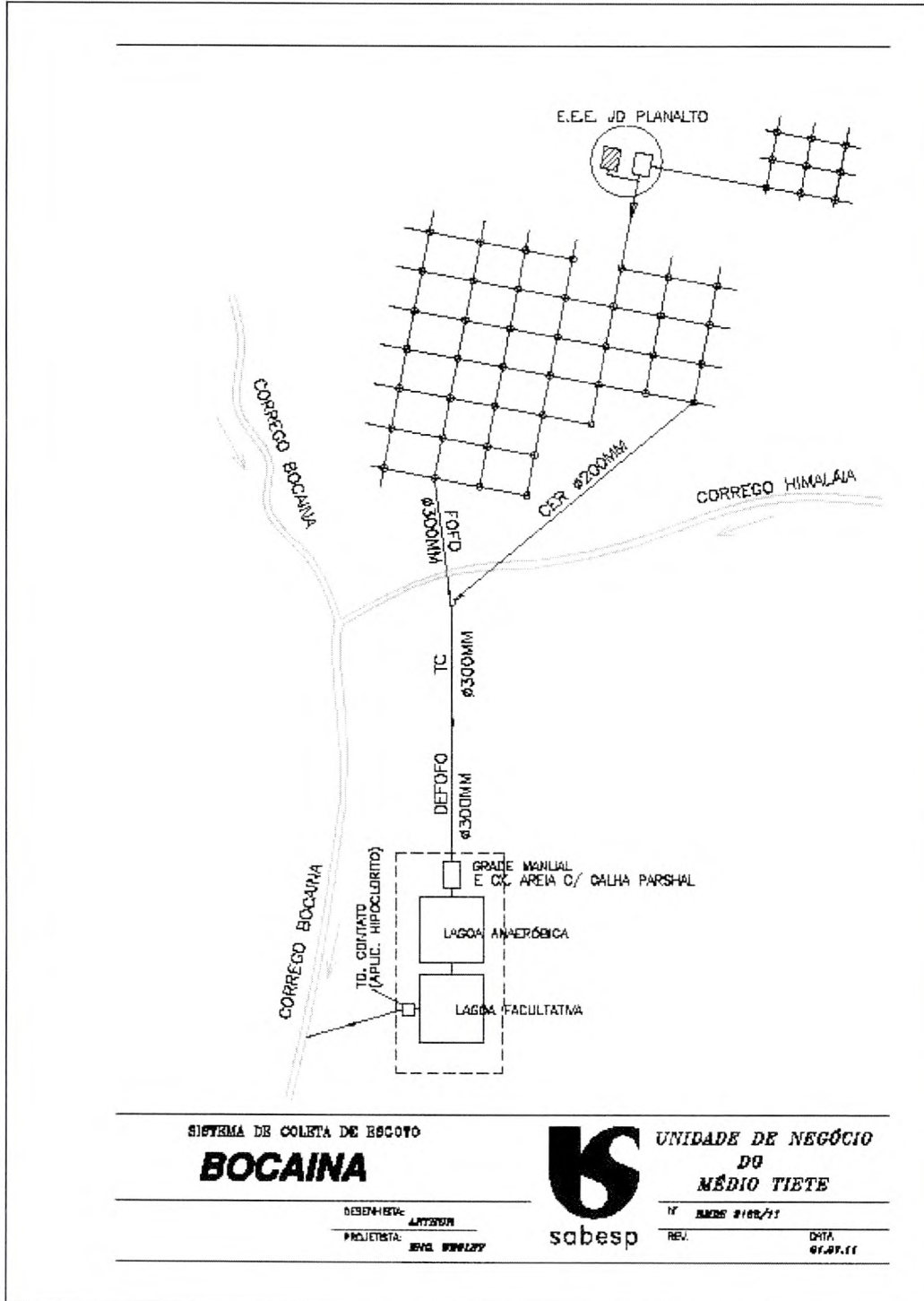
Figura 5 - Sistema Sintético dos Esgotos Sanitários - Fonte SABESP
